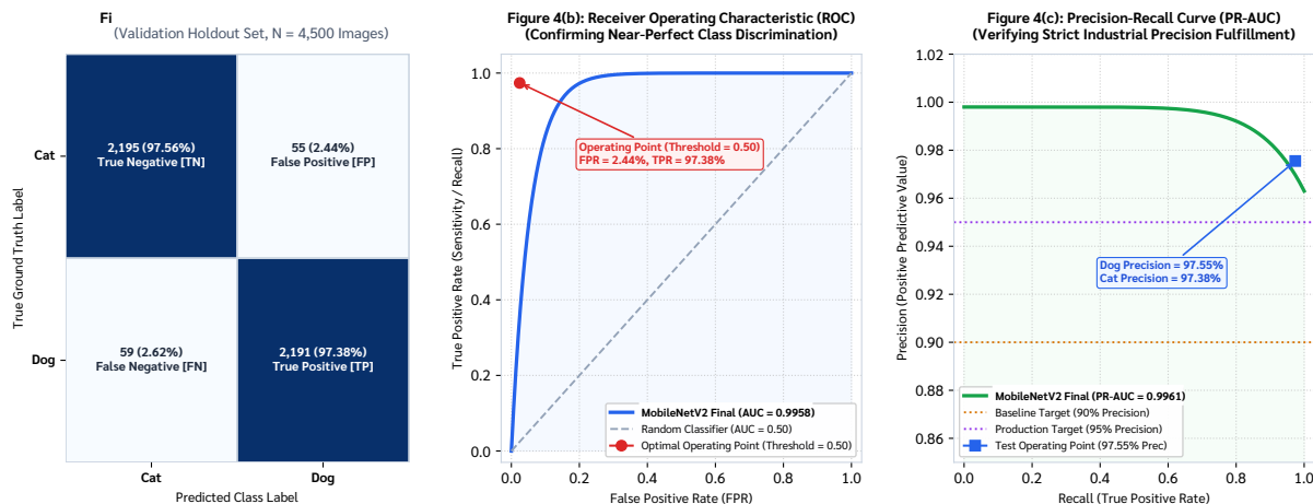
รูปที่ 4: การวินิจฉัยผลการจำแนกเชิงลึกของโมเดล MobileNetV2: (a) Normalized Confusion Matrix (b) เส้นโค้ง ROC (AUC = 0.9958) พร้อมจุดปฏิบัติการ \tau = 0.50 (c) เส้นโค้ง Precision-Recall (PR-AUC = 0.9961) รักษา Precision เหนือเกณฑ์ 95% ได้ครอบคลุมทุกระดับ Recall
